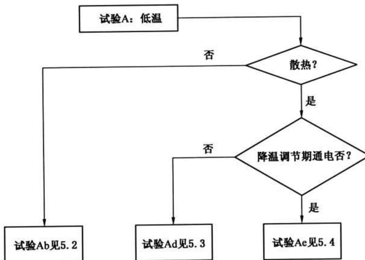
图1 试验A:低温试验方框图
